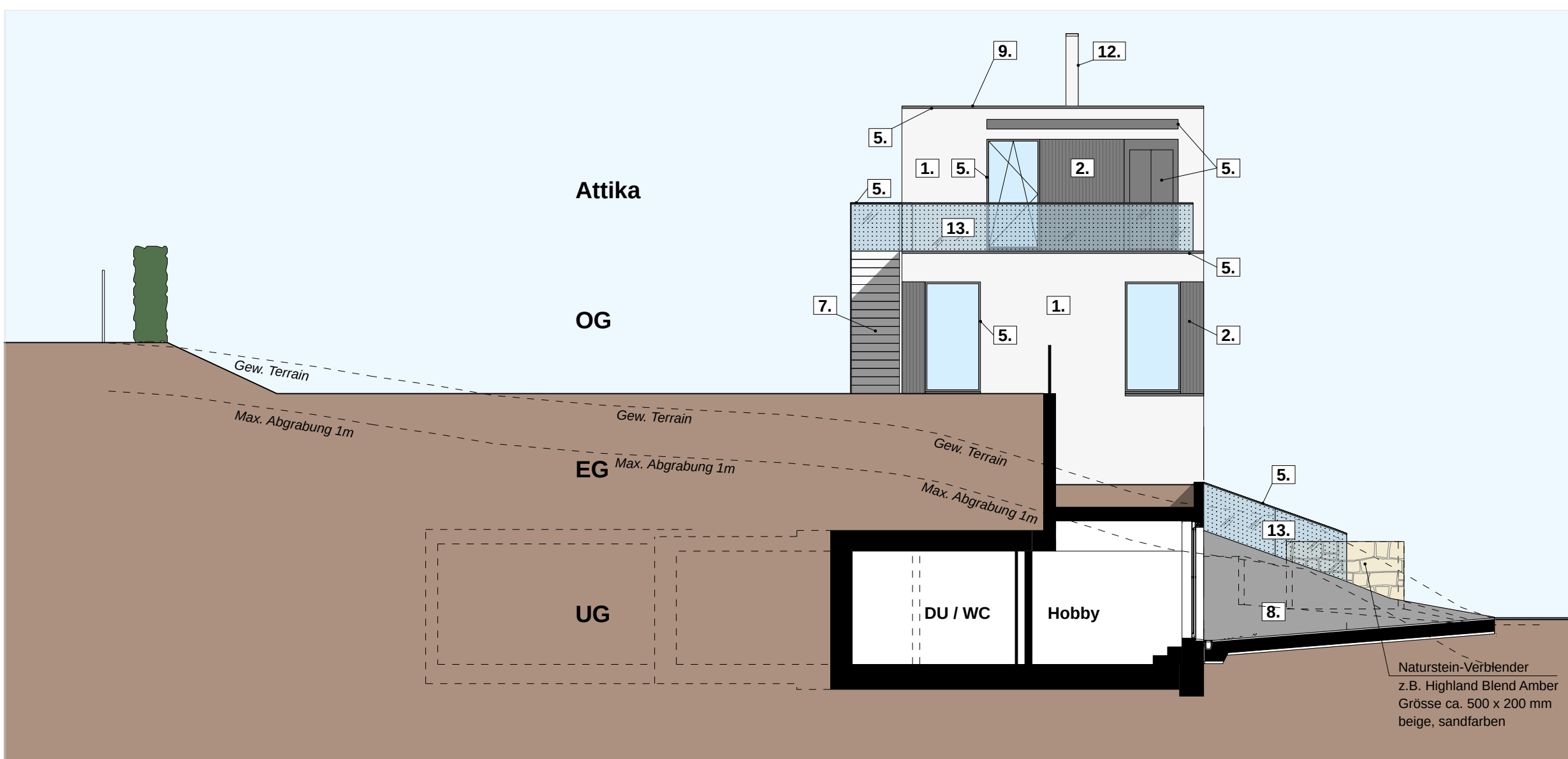
Westseite Haus B
