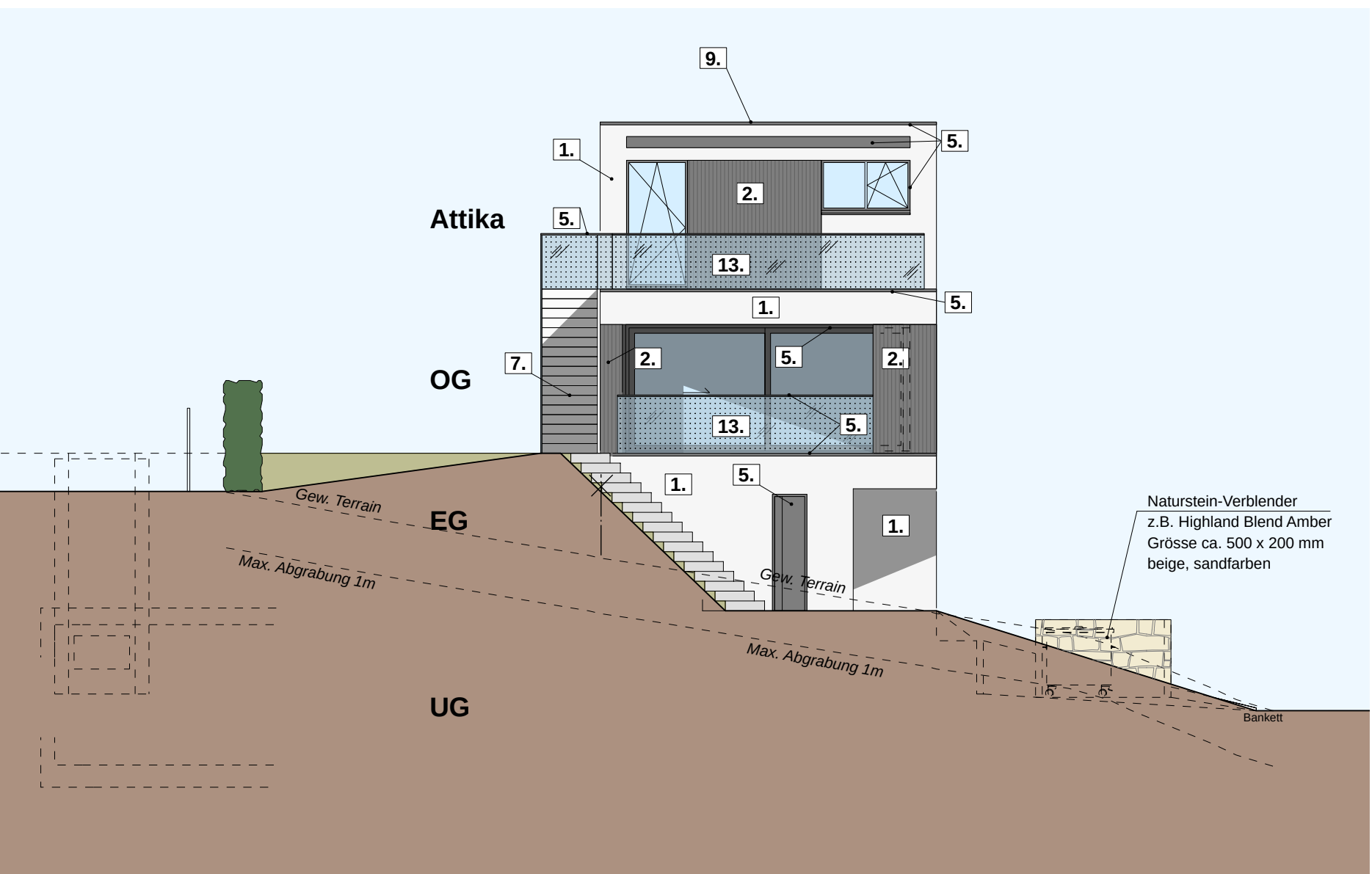
Westseite Haus A
