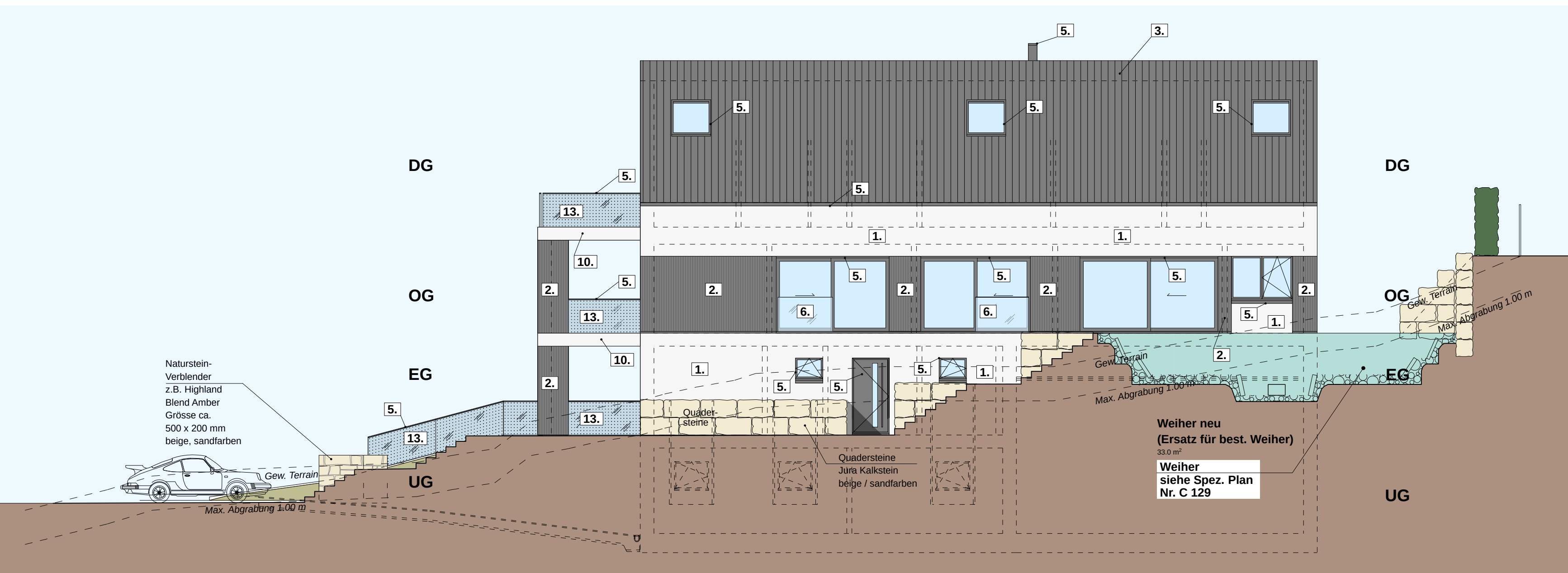
Ostseite Haus C
