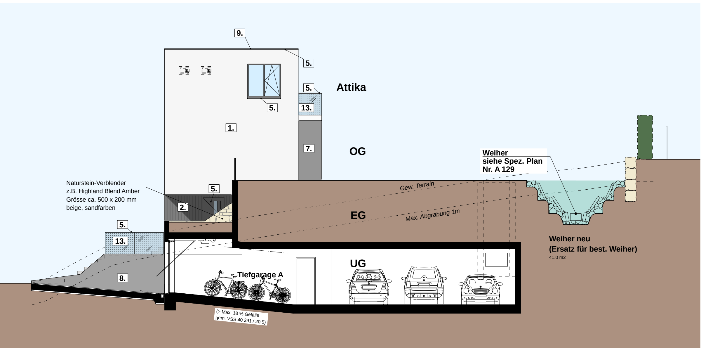
Ostseite Haus A
