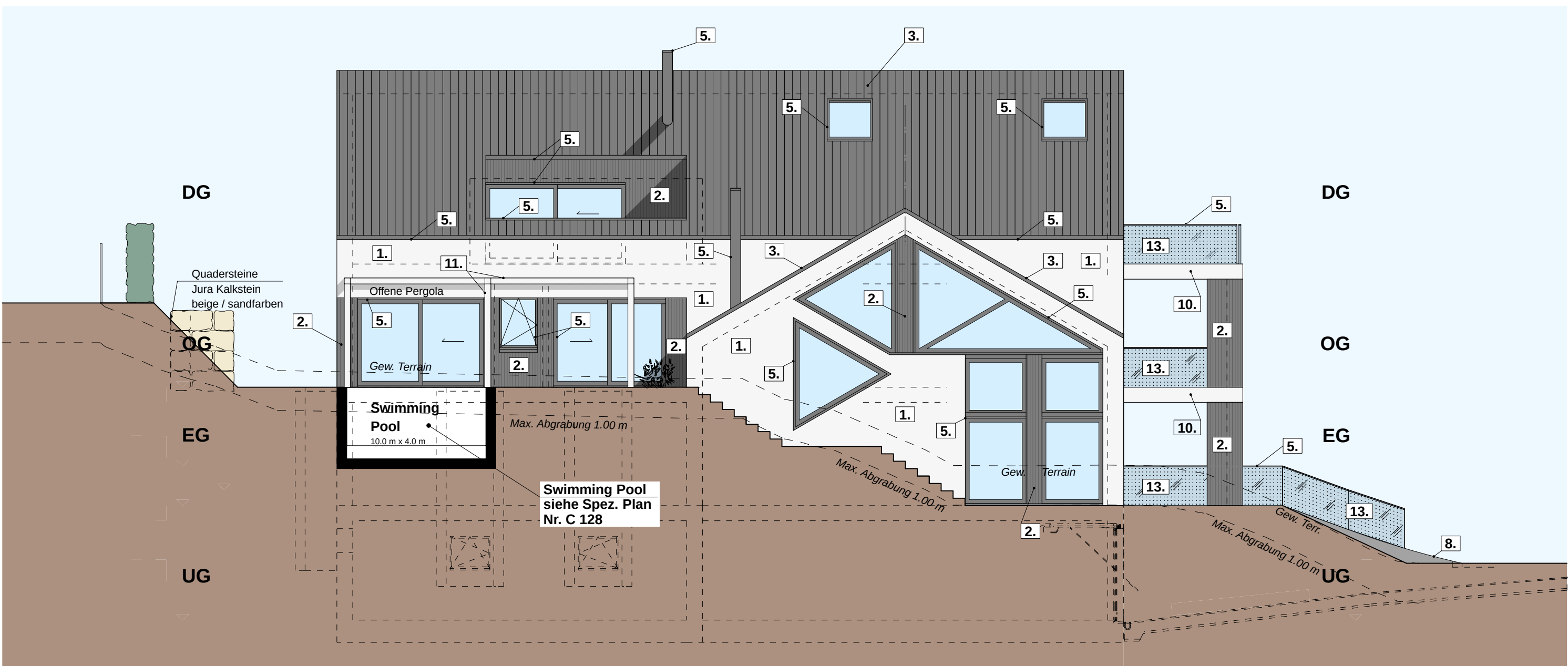
Westseite Haus C
