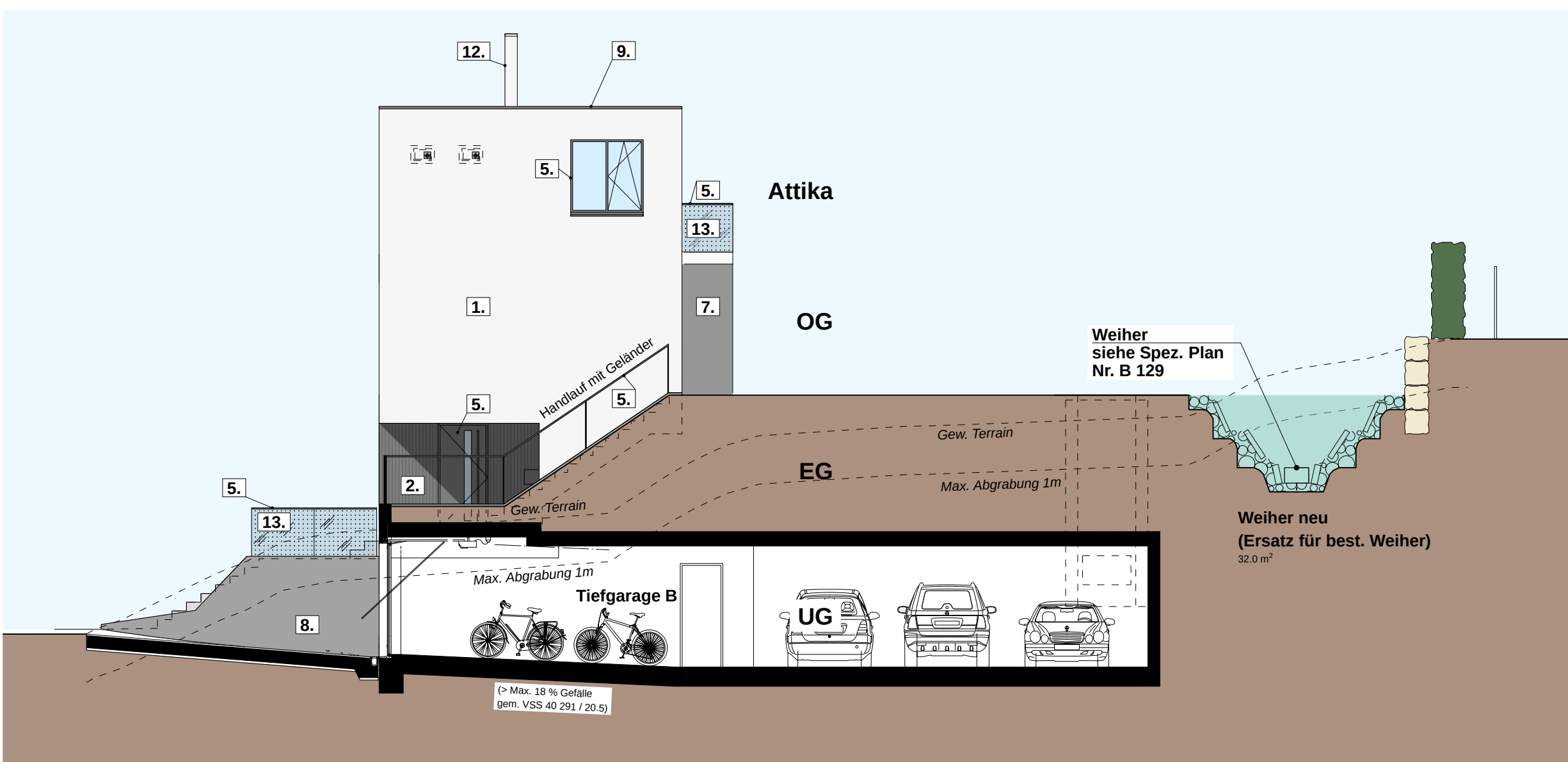
Ostseite Haus B
